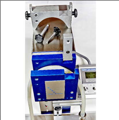
VAM- Abfüllköpfe VAM- filling heads
