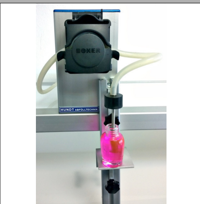
ECO1000 für kleine Volumen 0,5ml - 25ml ECO1000 for small volume 0,5cc -25cc
