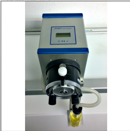
ECO3000 mit Düsen/Flaschen Stativ ECO3000 with nozzle/bottle stand
